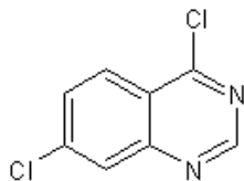
4,7-Dichloroquinazoline
