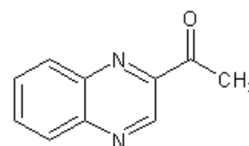
2-Acetylquinazoline
