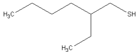
2-Ethyl-1-hexanethiol
