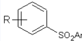
Arylsulphones
