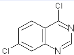
4,7-Dichloroquinazoline
