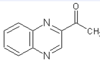
2-Acetylquinoxaline
