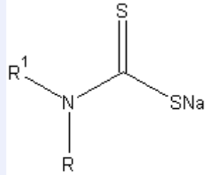
Dithiocarbamates
